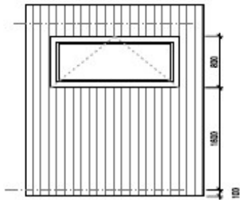
boční pohled
